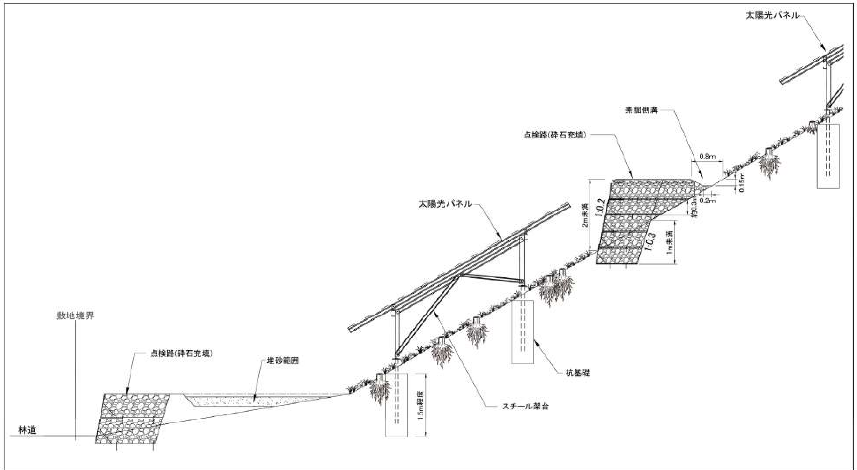
圖 1.8-2 太陽光設備断面模式圖
