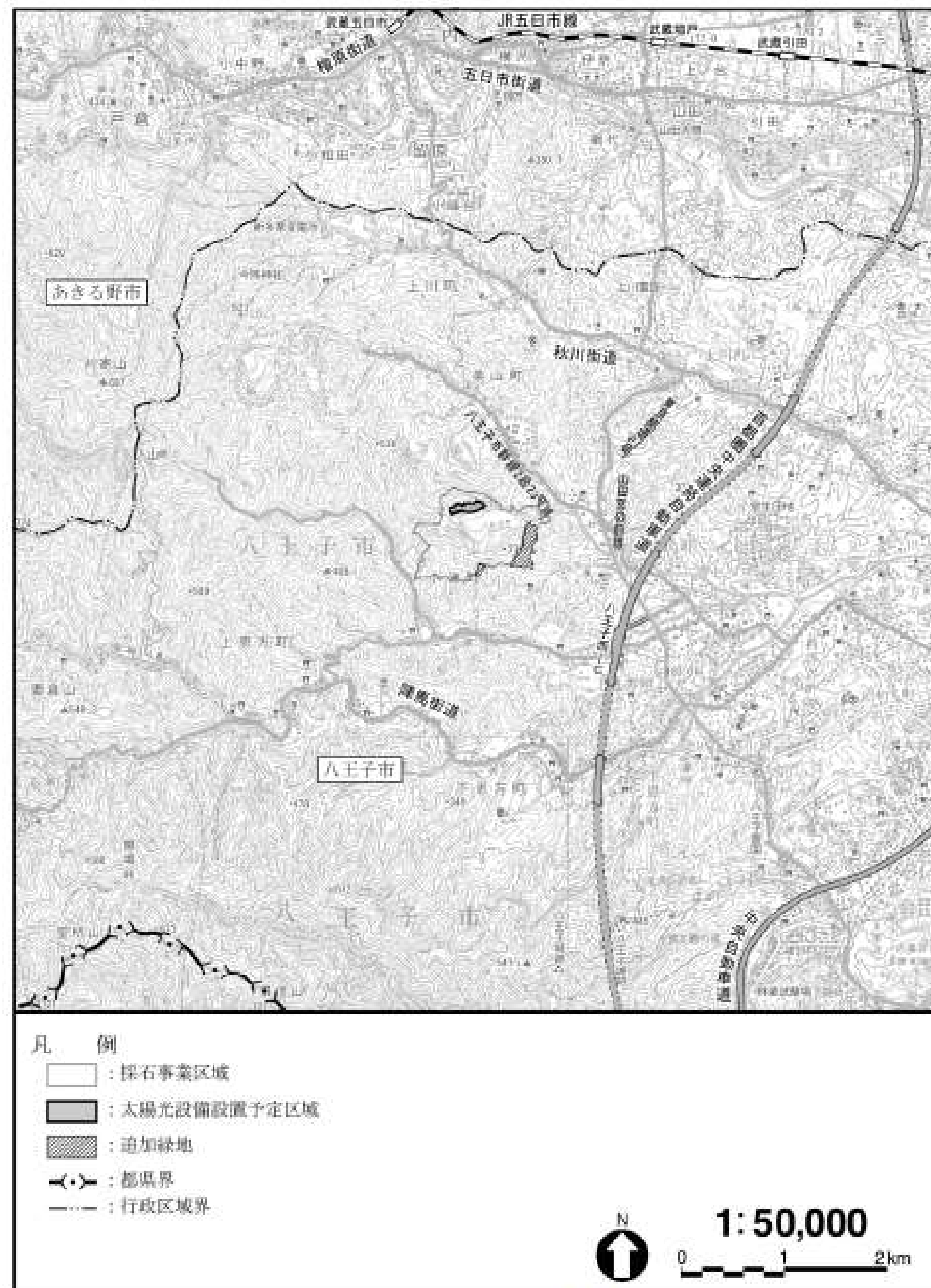
図 1.2-1 採石事業区域及び太陽光設備設置予定区域等位置図
