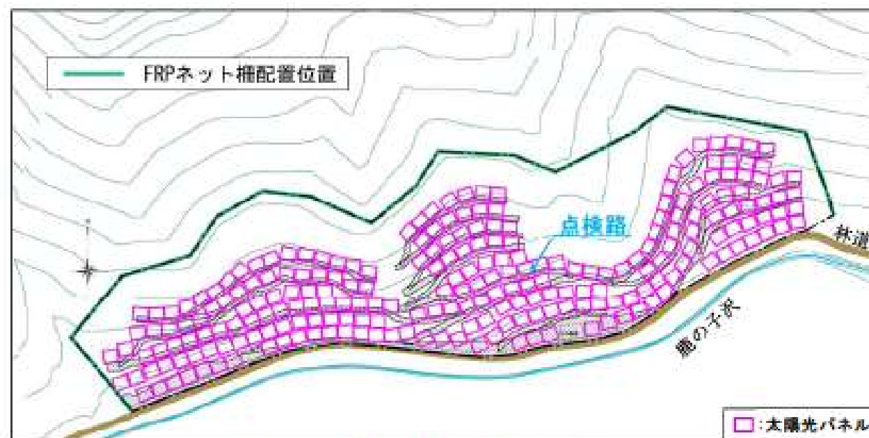
図 1.9-2 FRP ネット柵配置位置図
