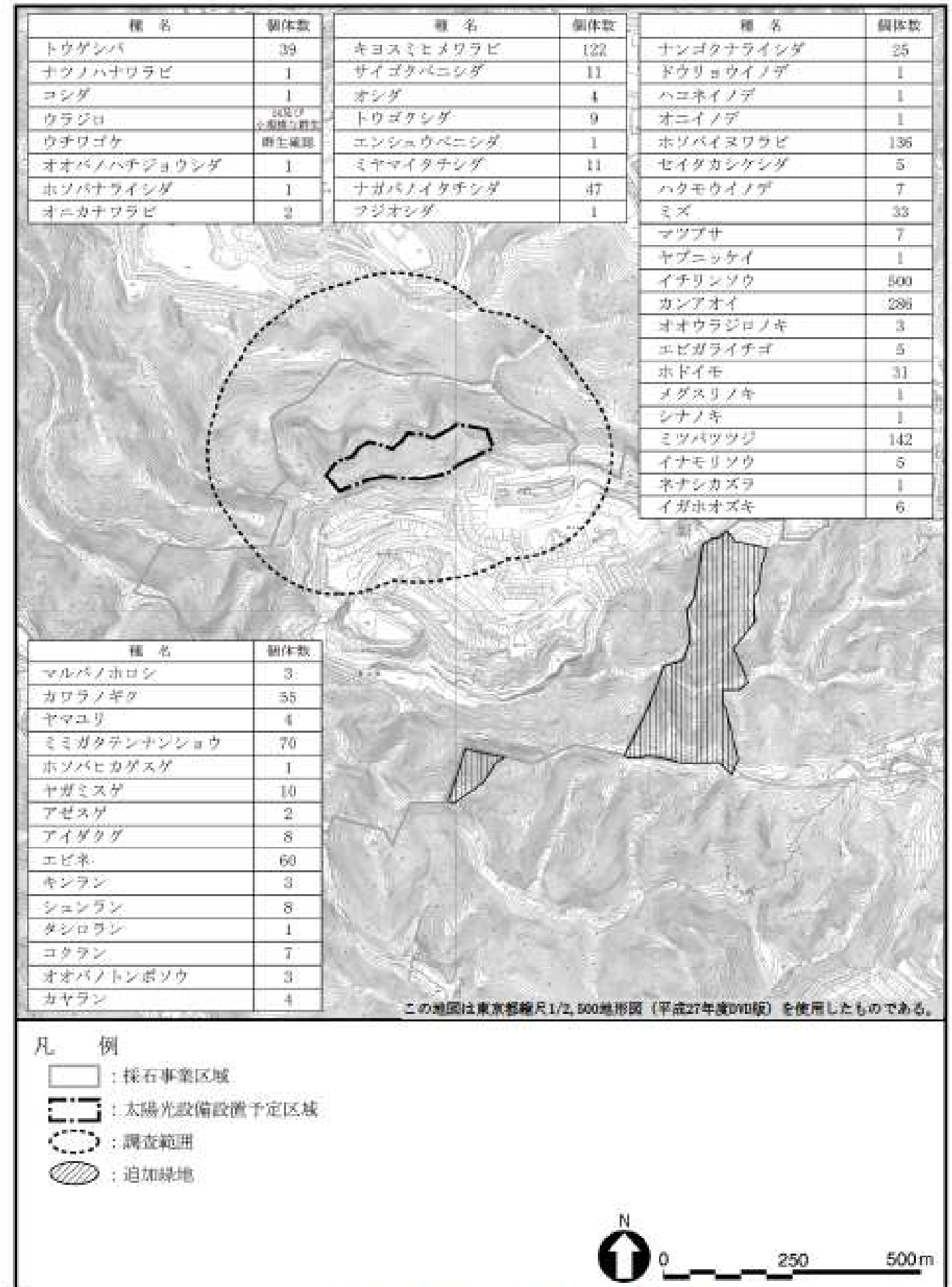
図 2.2.1-1 注目される植物種確認地点位置図
