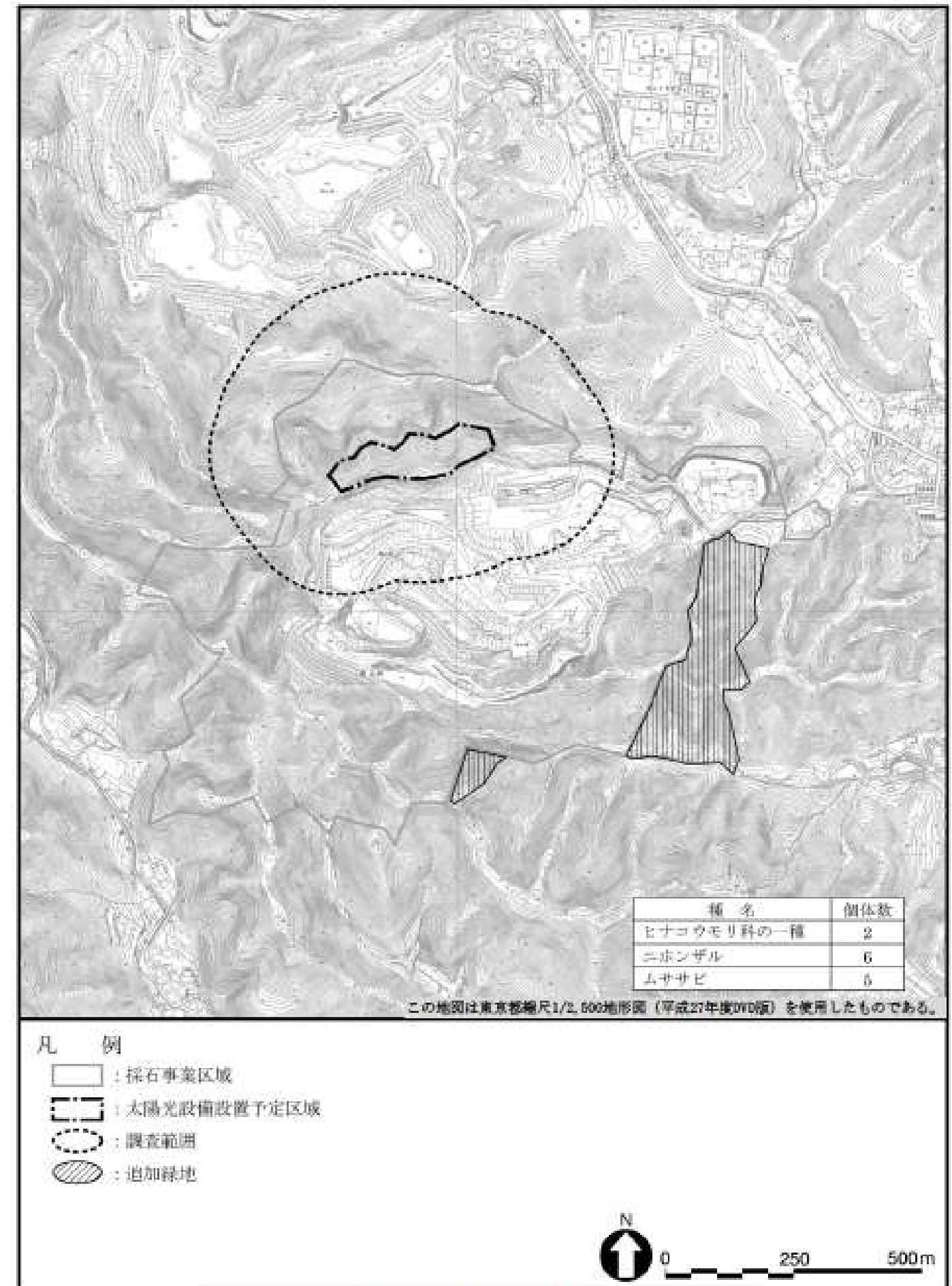
図2.2.2-1 注目される種（ほ乳類）の確認地点
