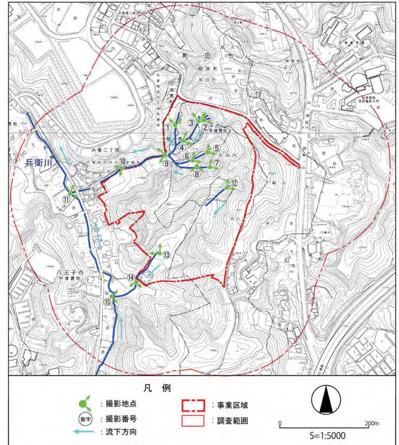
図 2-2-2-1 水系位置図
