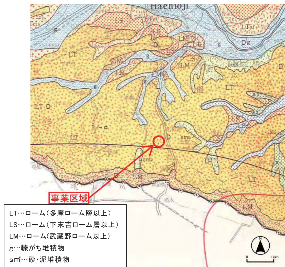
図 2-2-1-2 事業区域周辺の表層地質図
