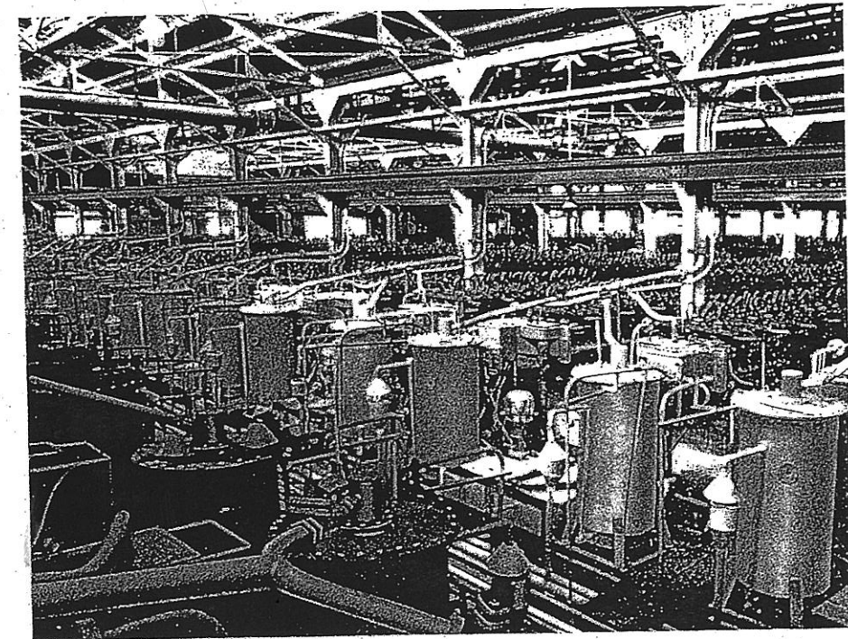
水銀法電解室
