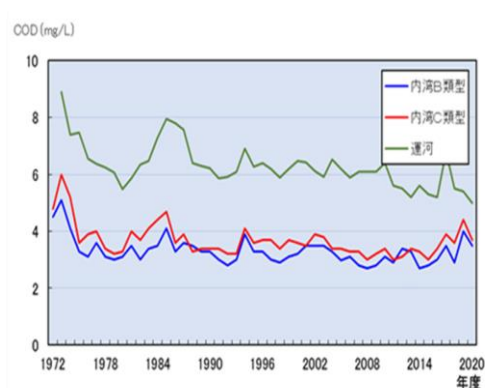
東京湾のCODの経年変化(年度平均値)
