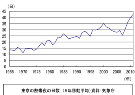
図表 5-4-11 東京の熱帯夜の日数の推移
