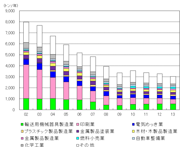
図表 5-4-10 環境への排出量の推移（都内）
