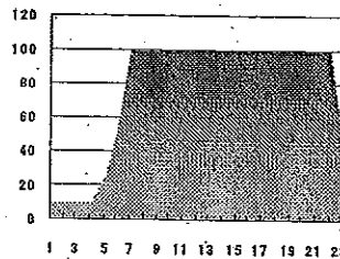
図2: 飲食店における電力需要カーブの事例
