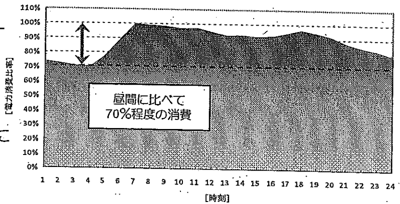
図2：平均的なホテル・旅館における電力需要カーブのイメージ 出典：資源エネルギー庁推計
