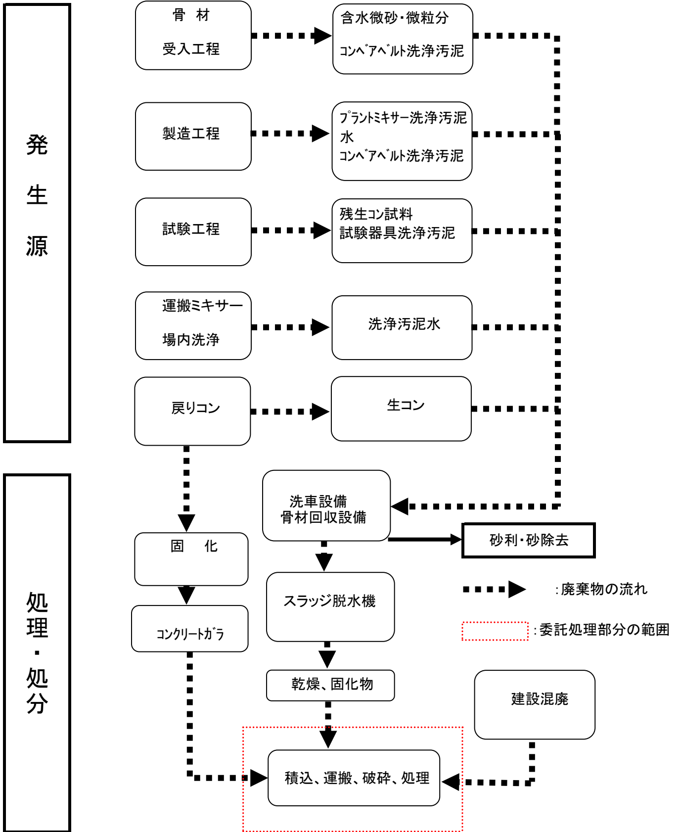
図③ 廃棄物処理フロー図
