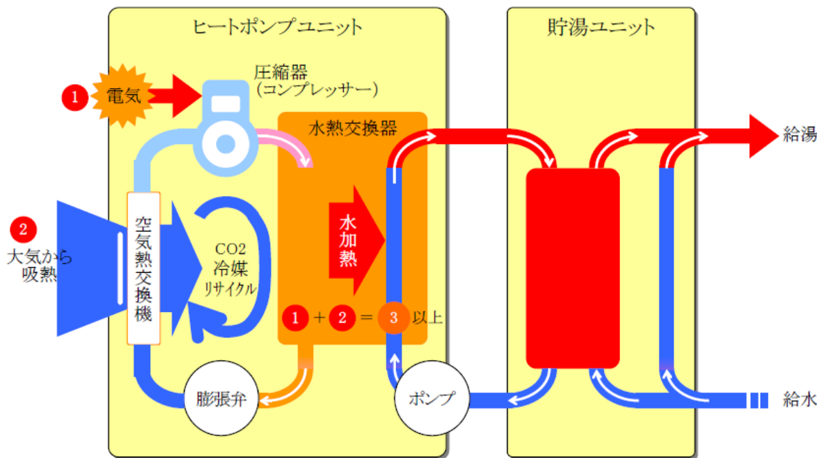
自然冷媒ヒートポンプ給湯器
