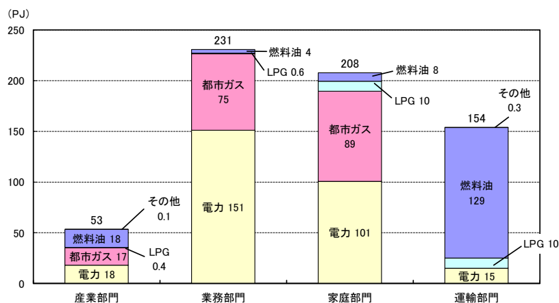
図 2-2 東京都における最終エネルギー消費の部門別状況（2014年度）
