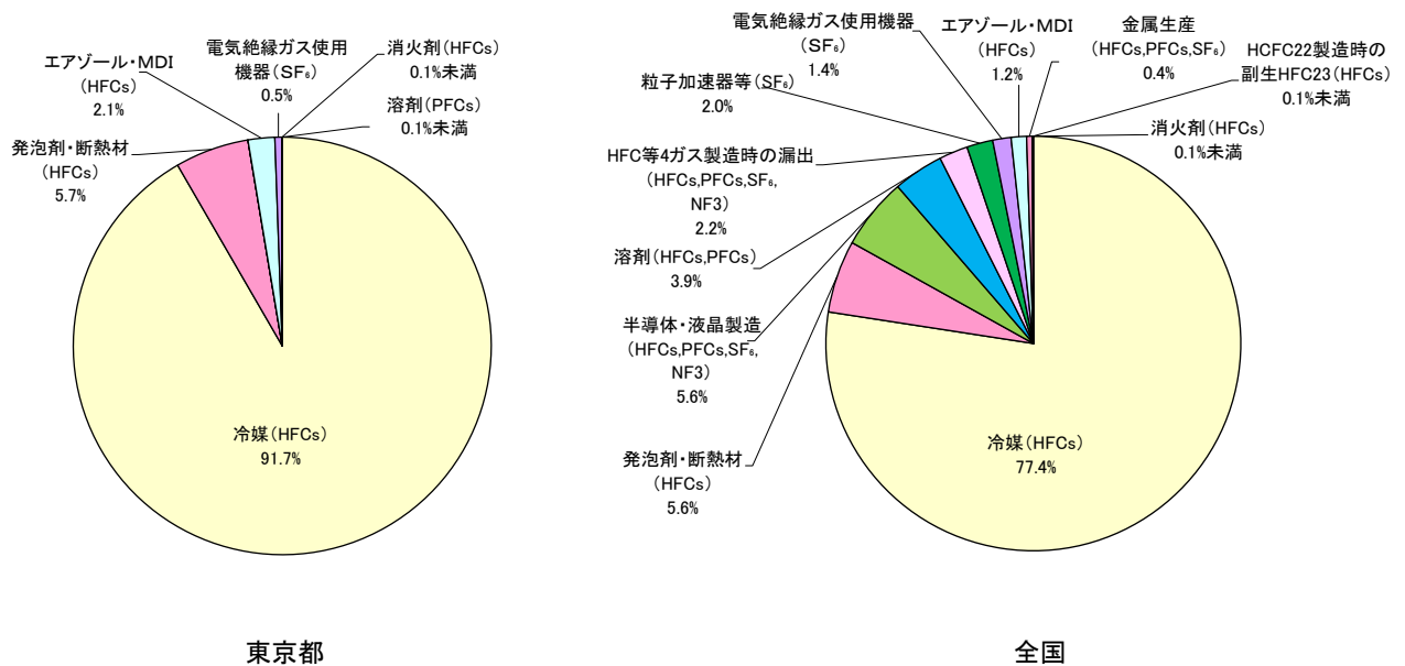
図 3-25 東京都と全国のHFC等4ガス排出構成比（2014年度）
