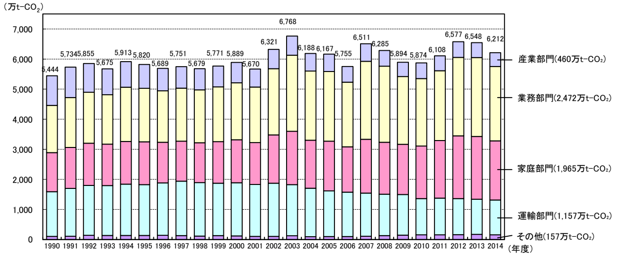
図 3-6 東京都における総 CO 2 排出量（部門別）の推移【変動ケース】
