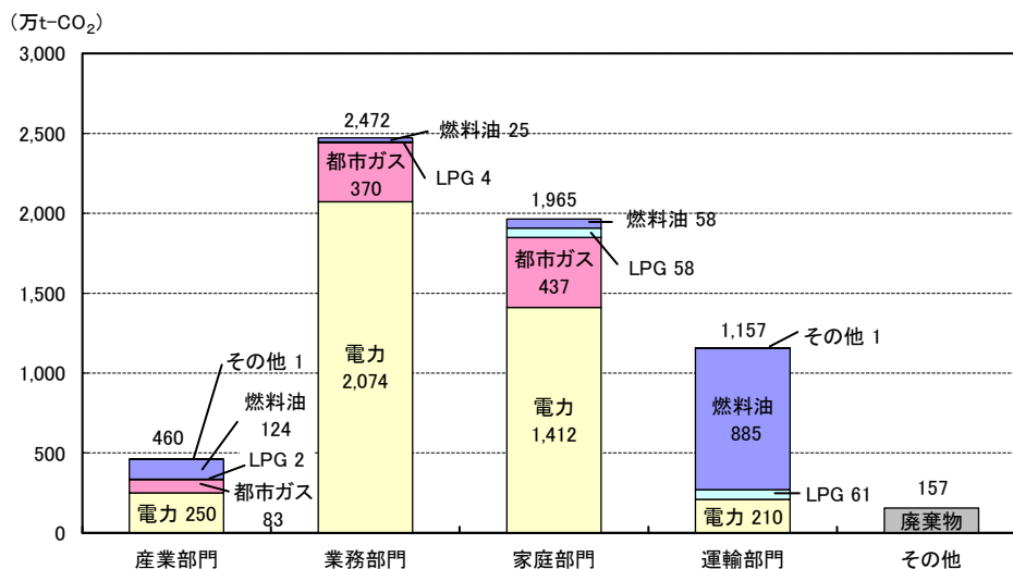
図 3-5 東京都における二酸化炭素排出量の部門別状況（2014年度）【変動ケース】
