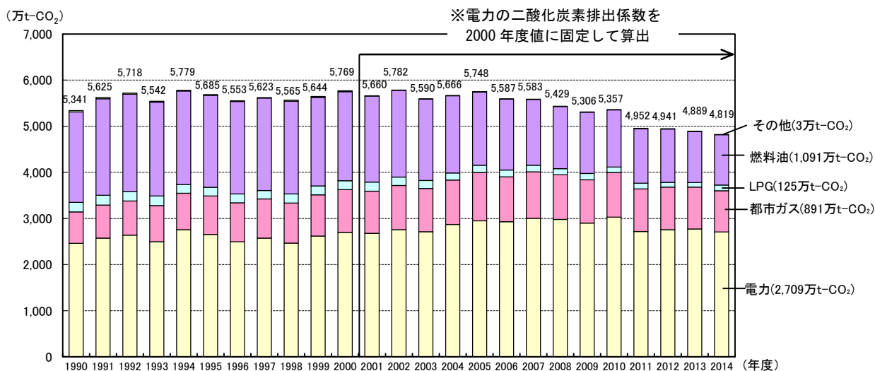
図 3-15 東京都におけるエネルギー起源 CO 2 排出量（燃料種別）の推移【固定ケース】
