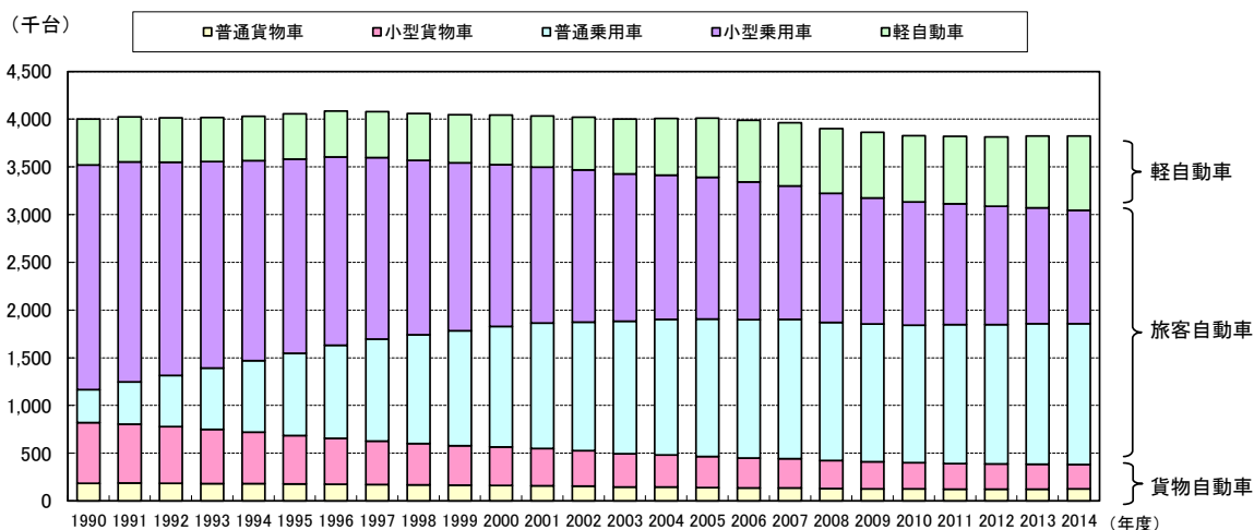
図 2-33 東京都の自動車保有台数の推移
