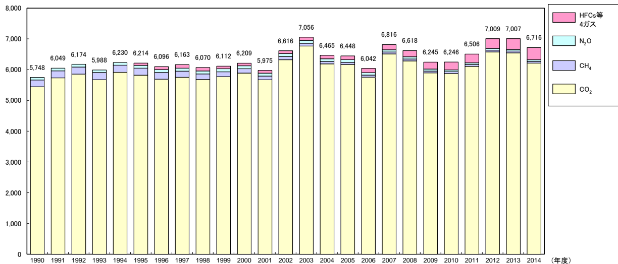
図 3-2 東京都における温室効果ガス総排出量の推移【変動ケース】
