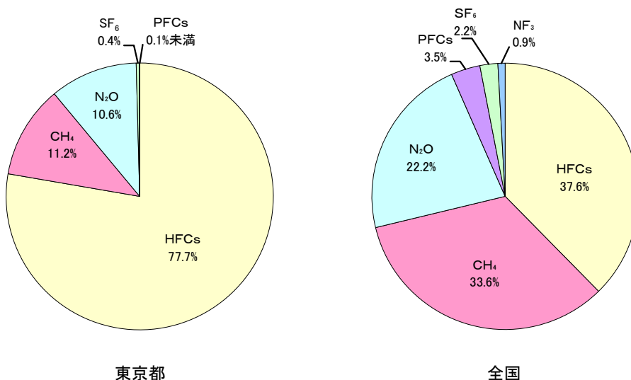
図 3-22 東京都と全国のその他の温室効果ガス排出構成比 (2014年度)
