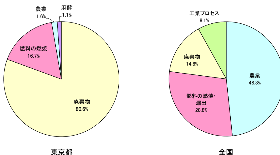
図 3-24 東京都と全国の一酸化二窒素排出構成比（2014年度）
