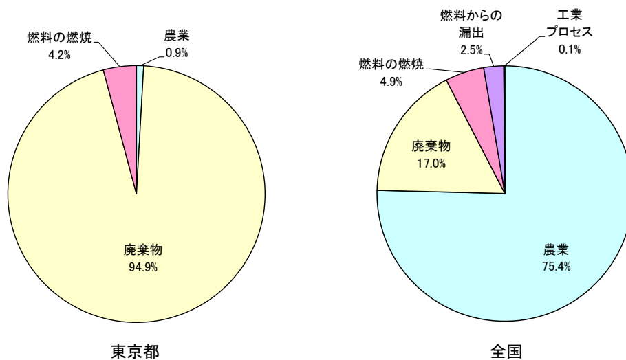
図 3-23 東京都と全国のメタン排出構成比（2014年度）
