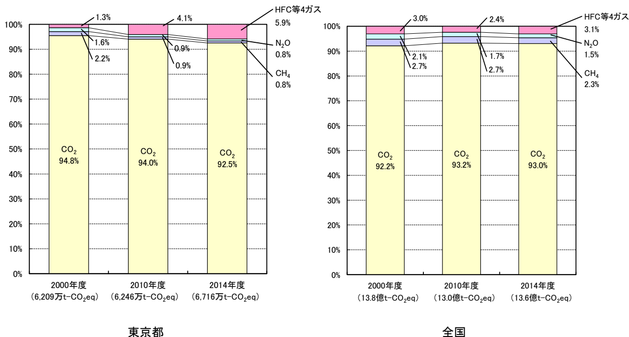
図 3-3 東京都と全国の温室効果ガス別排出構成比【変動ケース】
