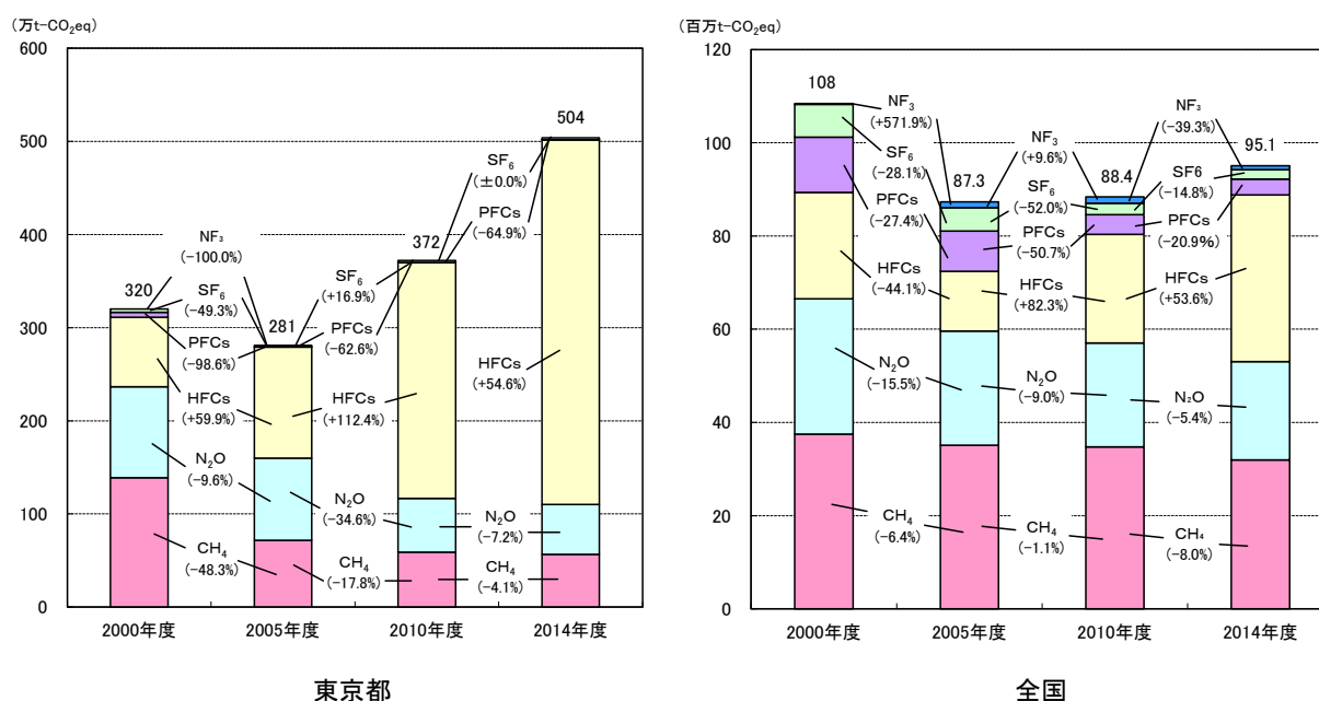
図 3-21 東京都と全国のその他の温室効果ガス別排出量の伸び
