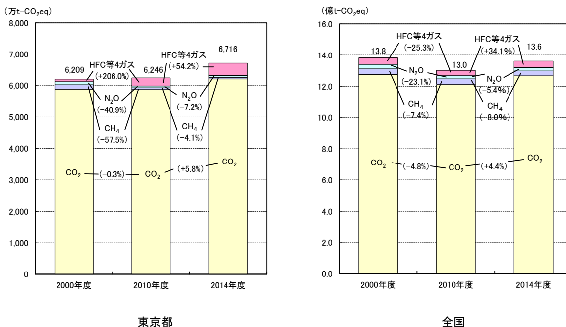
図 3-4 東京都と全国の温室効果ガス別排出量の伸び【変動ケース】
