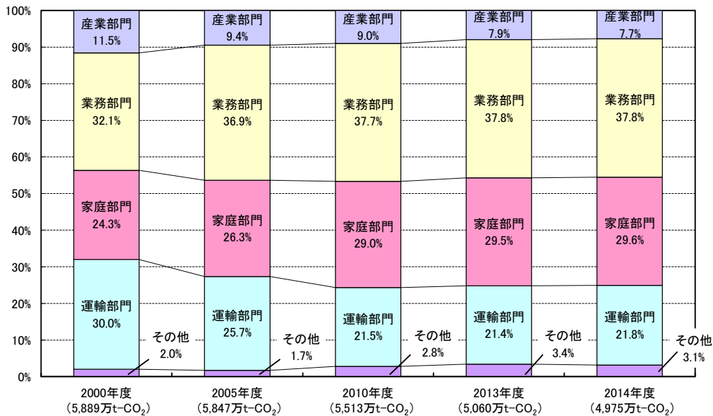
図 3-14 東京都における総 CO 2 排出量（部門別）の構成比【固定ケース】
