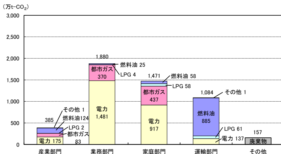
図 3-12 東京都における二酸化炭素排出量の部門別状況（2014年度）【固定ケース】
