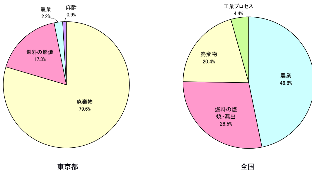
図 3-20 東京都と全国の一酸化二窒素排出構成比（2018年度）
