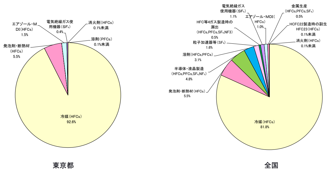
図 3-21 東京都と全国のHFC等4ガス排出構成比（2018年度）
