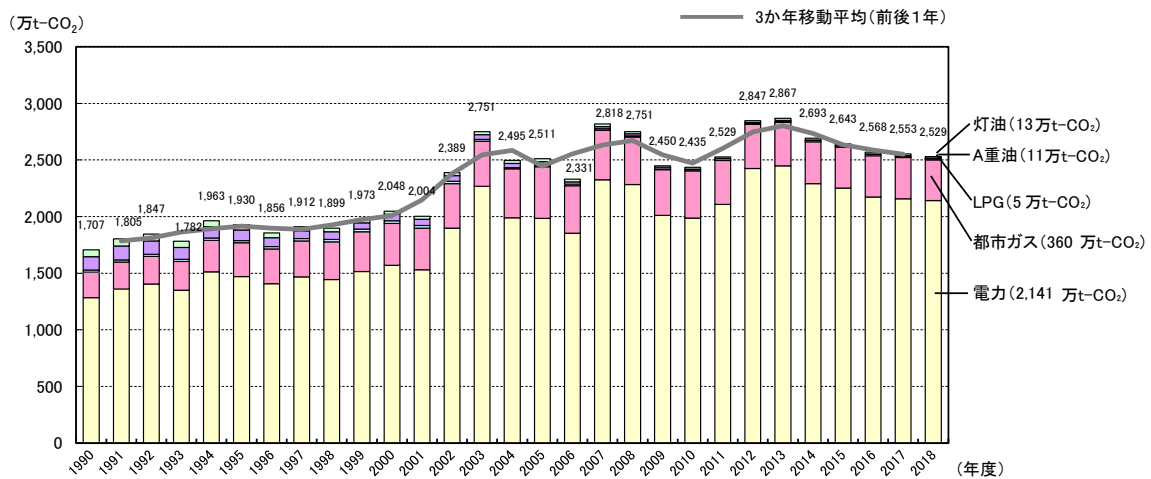
図 3-14 業務部門の二酸化炭素排出量の推移
