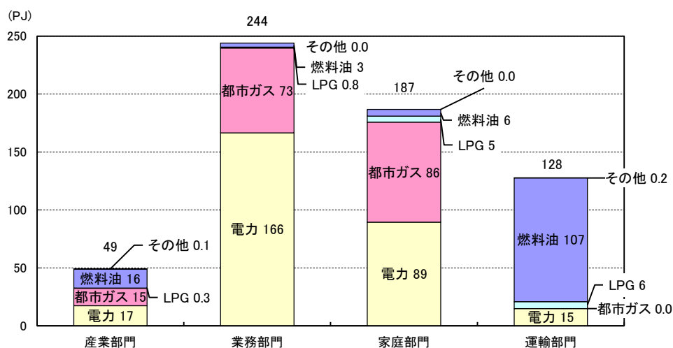
図 2-2 東京都における最終エネルギー消費の部門別状況（2018年度）
