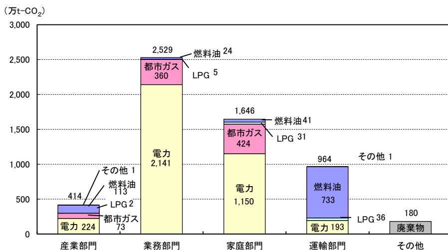
図 3-6 東京都における二酸化炭素排出量の部門別状況（2018年度）
