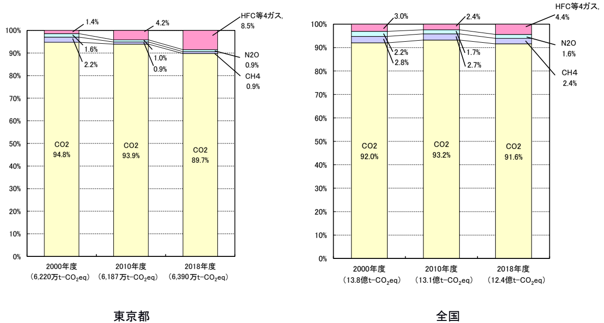
図 3-4 東京都と全国の温室効果ガス別排出構成比
