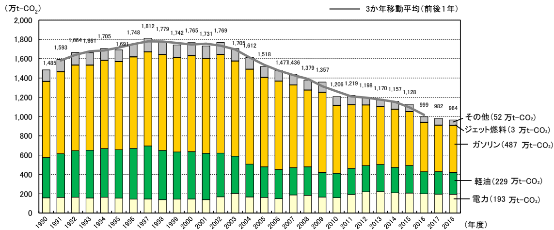
図 3-16 運輸部門の二酸化炭素排出量の推移
