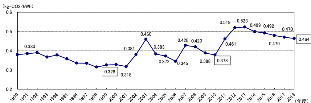
図 3-1 電力の二酸化炭素排出係数の推移
