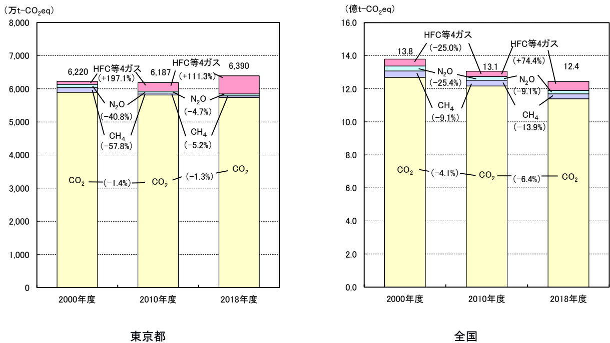
図 3-5 東京都と全国の温室効果ガス別排出量の伸び
