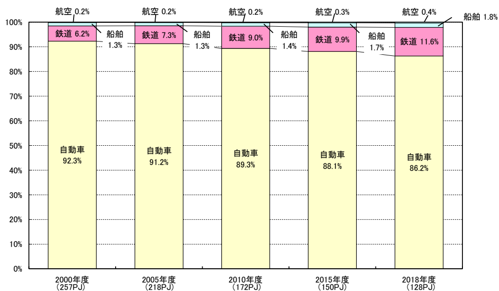
図 2-29 運輸部門の最終エネルギー消費（運輸機関別）の推移
