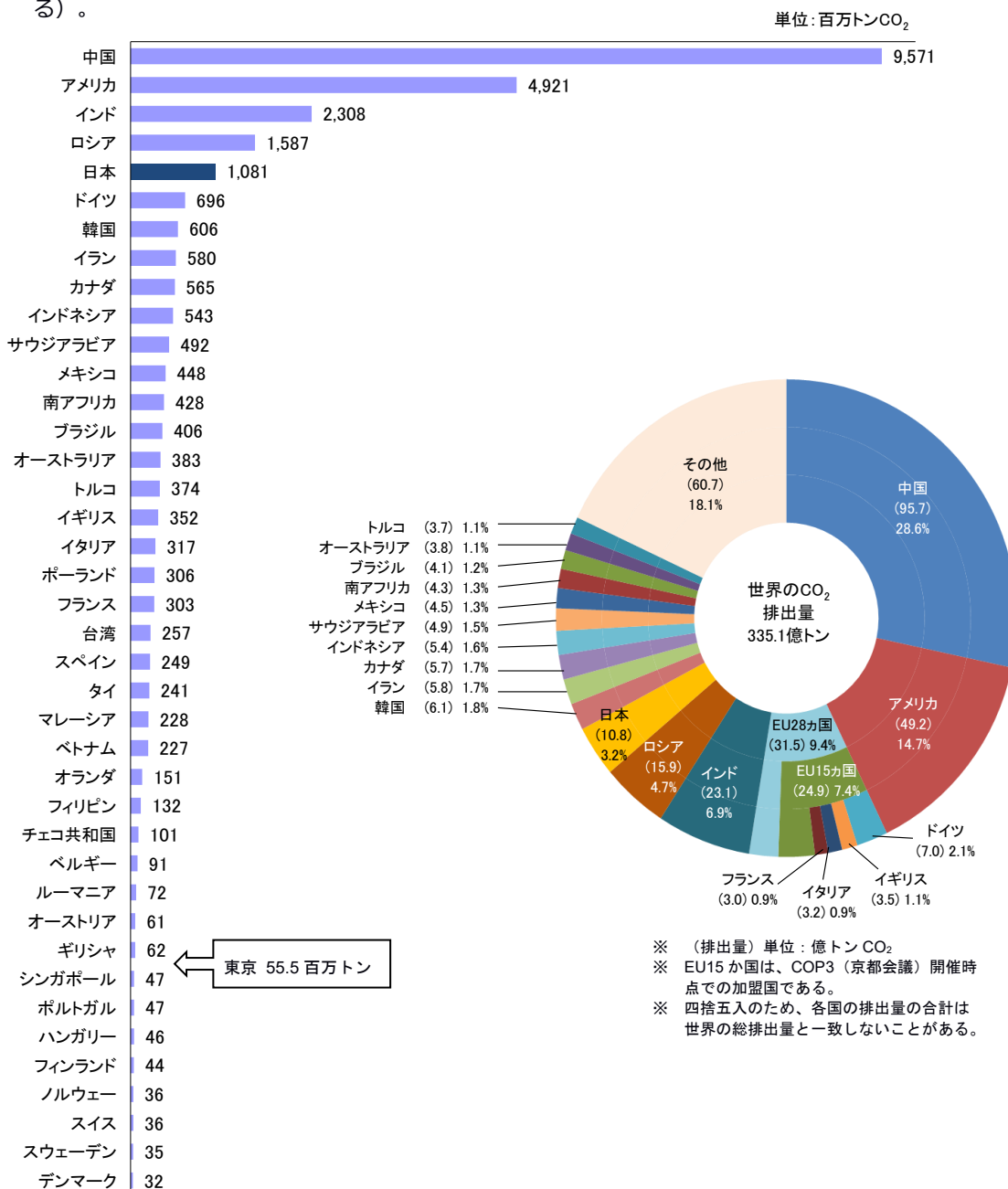
図 1-1 国別エネルギー起源 CO 2 排出量 (2018 年)
