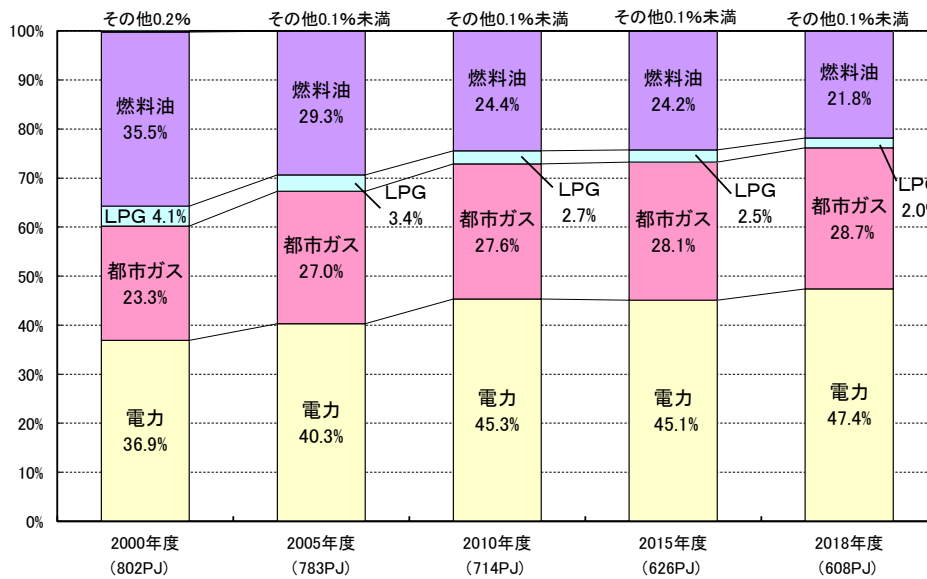
図 2-5 東京都における最終エネルギー消費（燃料種別）の推移
