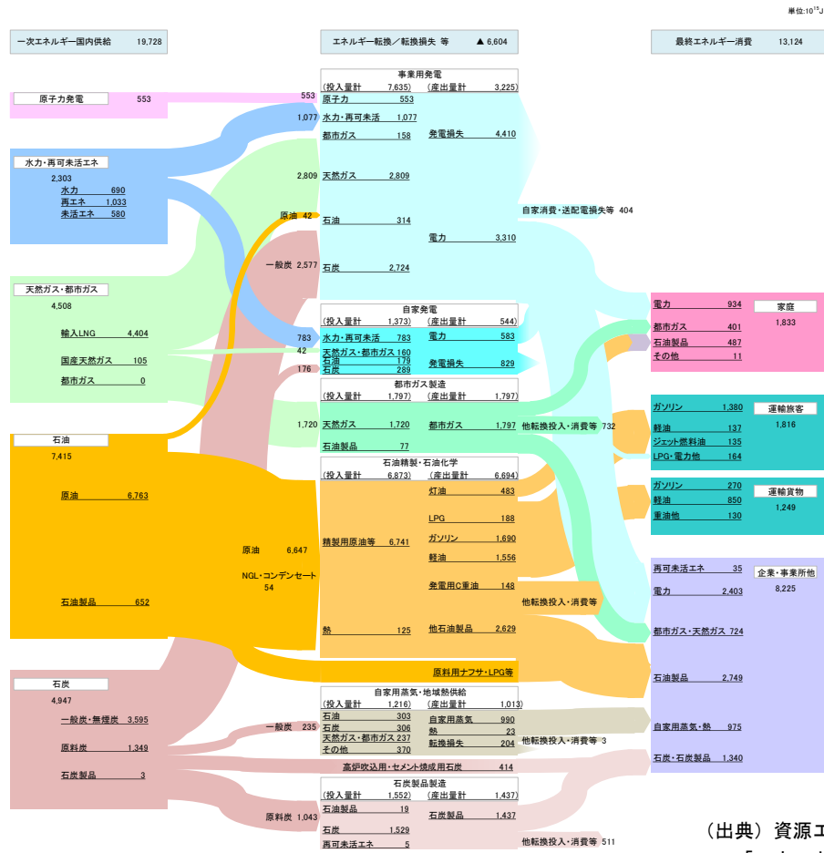
図 2-1 国内のエネルギーバランス・フロー概要 (2018 年度)
