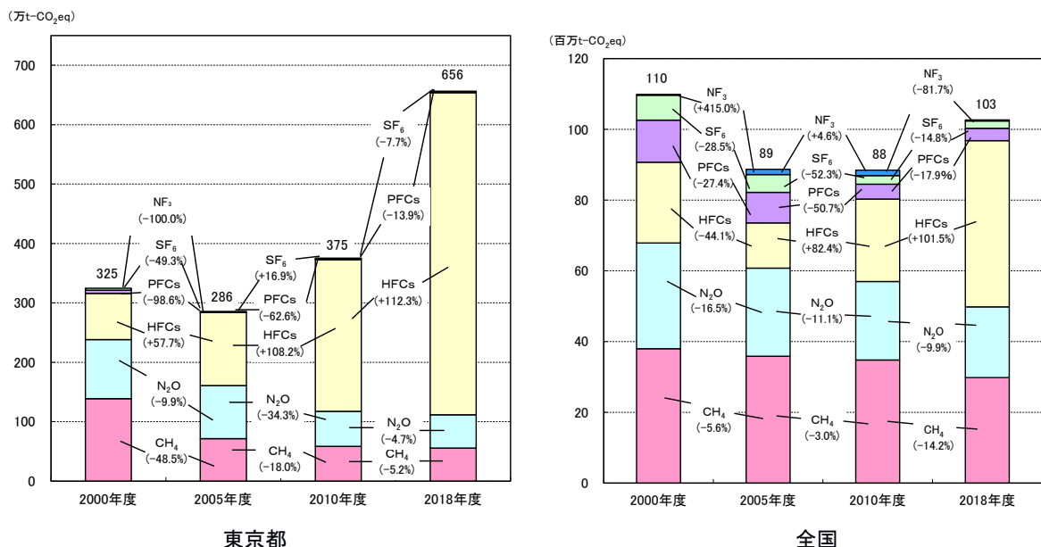
図 3-17 東京都と全国のその他の温室効果ガス別排出量の伸び
