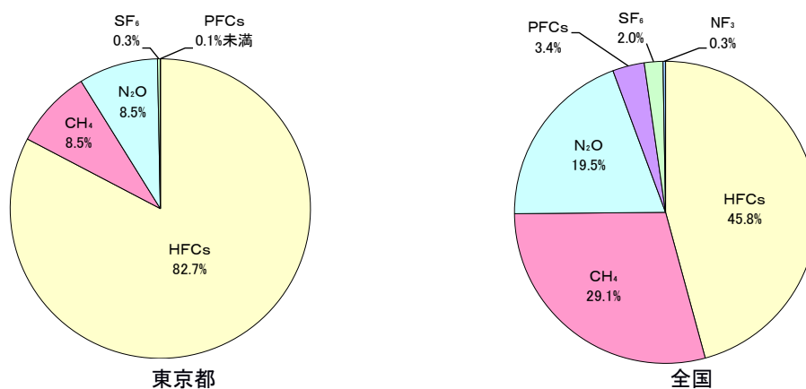
図 3-18 東京都と全国のその他の温室効果ガス排出構成比 (2018年度)
