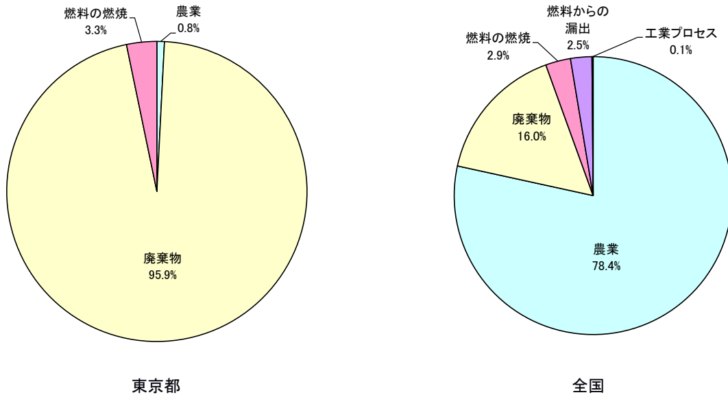
図 3-19 東京都と全国のメタン排出構成比（2018年度）
