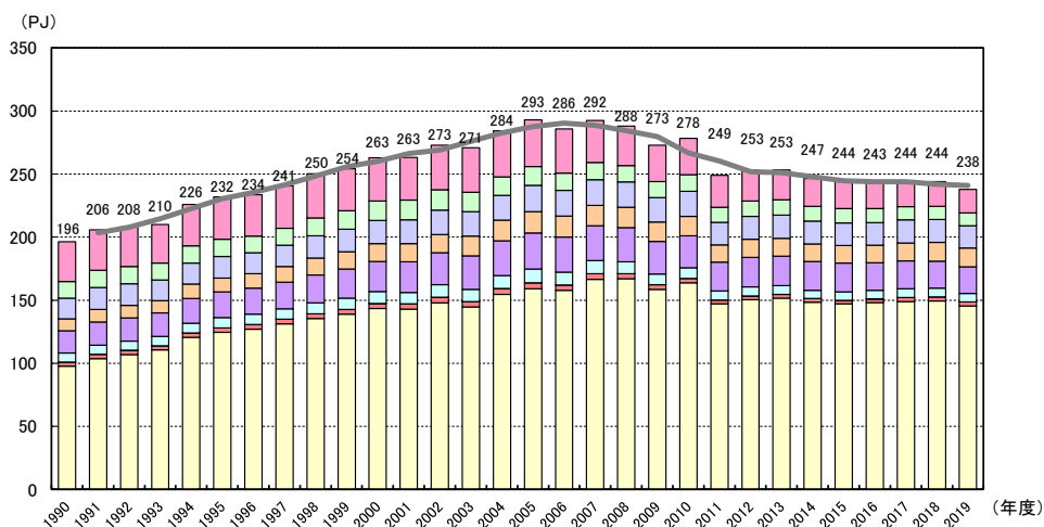
図 2-13 業務部門の最終エネルギー消費（建物用途別）の推移
